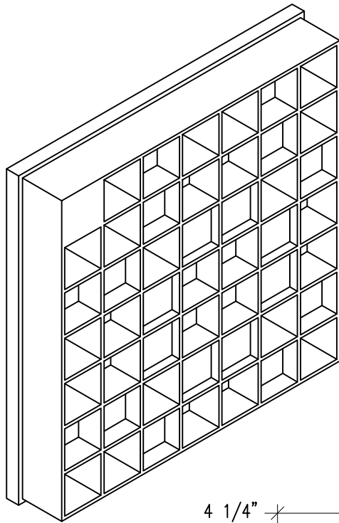
S.W. ISOMETRIC
